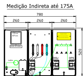
Medição Indireta até 175A
